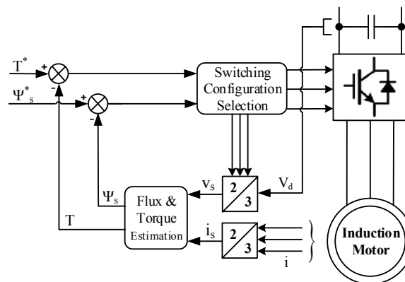
شکل ۱: نمای کلی روش DTC.
