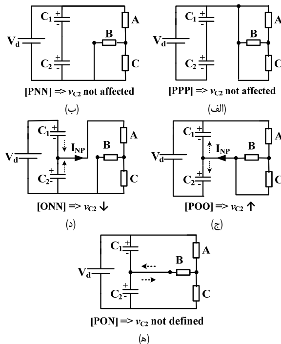
شکل ۶: اثر حالت‌های کلیدزنی بر انحراف ولتاژ نقطه خنثی، (الف) Zero Vector، (ب) Large Vector، (ج) P-Type Small Vector، (د) N-Type Small Vector، (ه) Medium Vector.
