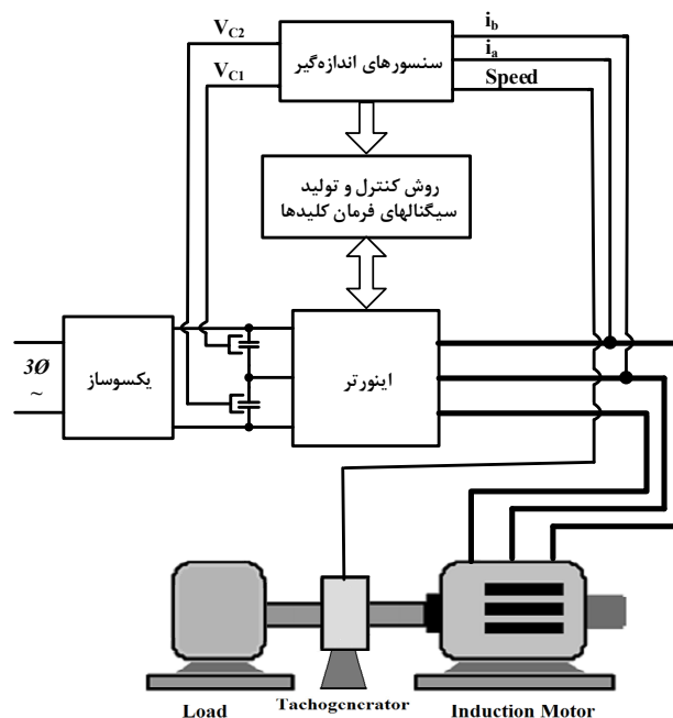
شکل ۹: شماتیک کلی سیستم کنترل سرعت.
