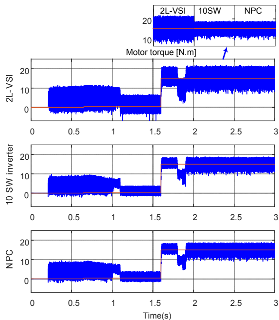
شکل ۱۱: گشتاور موتور.
