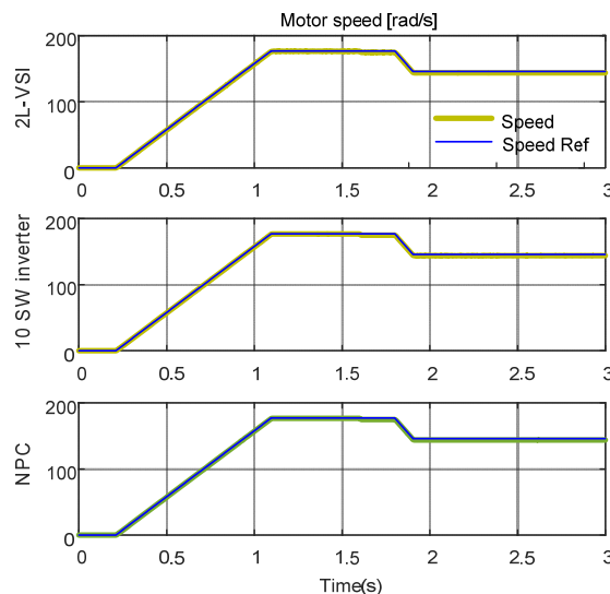
شکل ۱۰: سرعت موتور.
