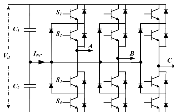
شکل ۲: اینورتر سه سطحی NPC.
