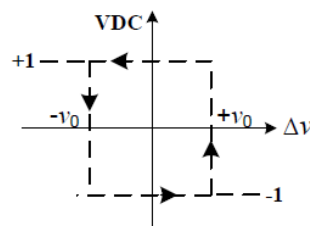
شکل ۷: کنترل گر هیستریز دوسطحی جهت کنترل انحراف ولتاژ.
