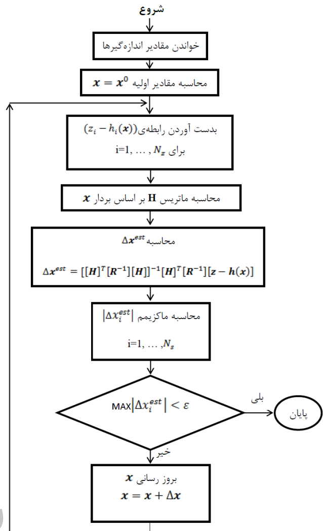
شکل ۱: روندنمای الگوریتم تکرار.
