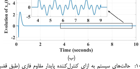
شکل ۱۲: ووردی کنترل کننده پایدار مقاوم فازی (طبق قضیه ۳). (الف) حالت i و (ب) حالت \omega .
