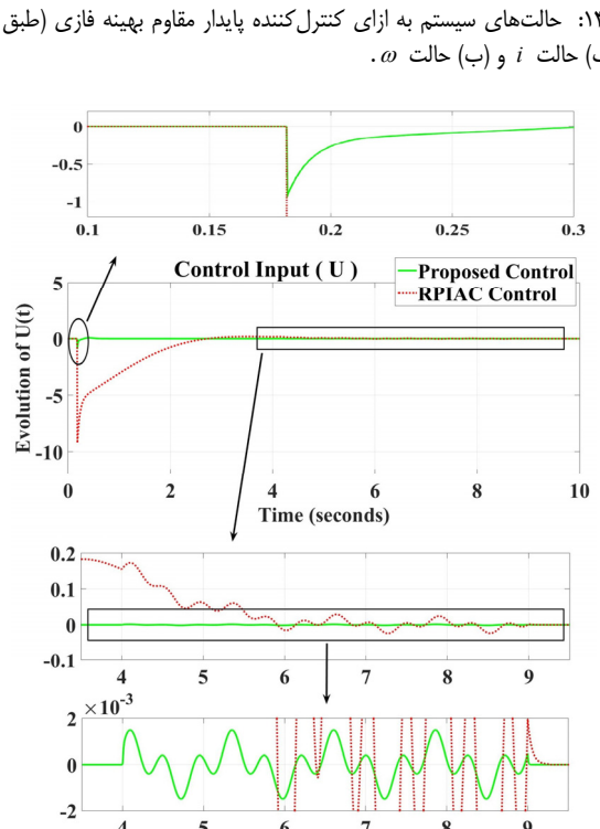
شکل ۱۵: مقایسه ورودی‌های کنترل کننده پایدار مقاوم بهینه فازی پیشنهادی و کنترل کننده [۱۸].
