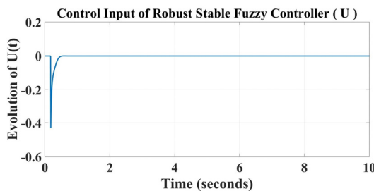
شکل ۶: ورودی کنترل کننده پایدار مقاوم فازی (طبق قضیه ۱).
