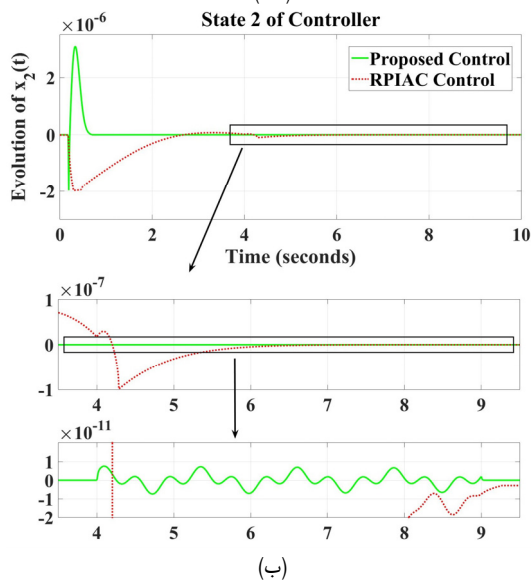
شکل ۱۶: مقایسه حالت‌های سیستم خودروی برقی به ازای کنترل کننده پایدار مقاوم بهینه فازی پیشنهادی و کنترل کننده [۱۸]، (الف) حالت i و (ب) حالت \omega .
