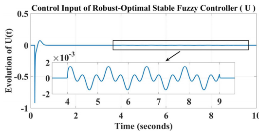
شکل ۱۰: ووردی کنترل کننده پایدار مقاوم فازی (طبق قضیه ۲). (الف) حالت i و (ب) حالت \omega .
