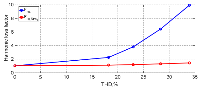
شکل ۵: ضریب هارمونیک بار برای تلفات جریان گردابی سیمپیچ و تلفات سرگردان ترانسفورماتور به ازای THD.
