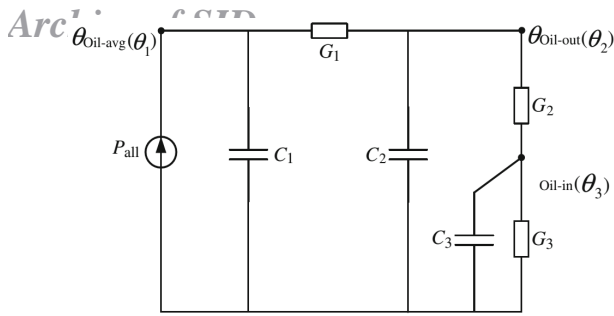
شکل ۳: یک نمونه مدار معادل حرارتی ساده شده [۲۵].
