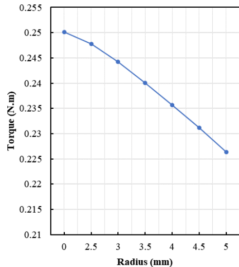
شکل ۱۸: مقایسه گشتاور میانگین موتور با رتور طراحی شده با اندازه شیارهای متفاوت.
