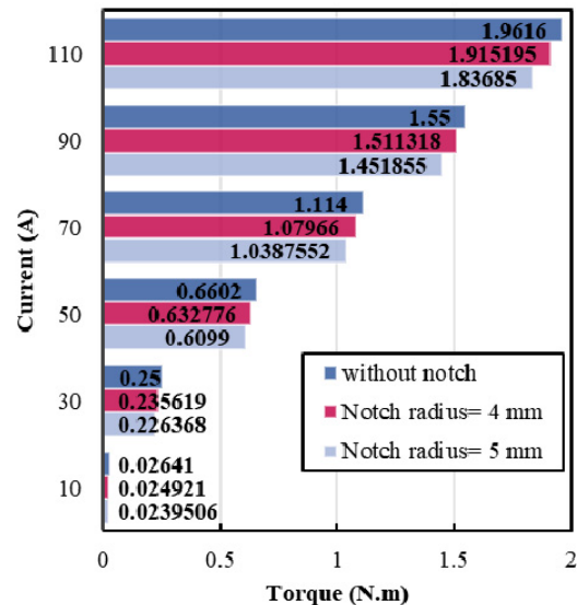
شکل ۲۰: مقایسه تلفات موتور با رتور طراحی شده با اندازه شیارهای متفاوت.
