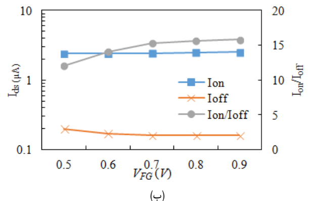
شکل ۹: نمودار تغییرات I_{on}/I_{off} (الف) بر حسب L_{FG} در V_{FG} = 0.7V و V_{DS} = 0.6V (ب) بر حسب V_{FG} در L_{FG} = 4nm و V_{DS} = 0.6V .
