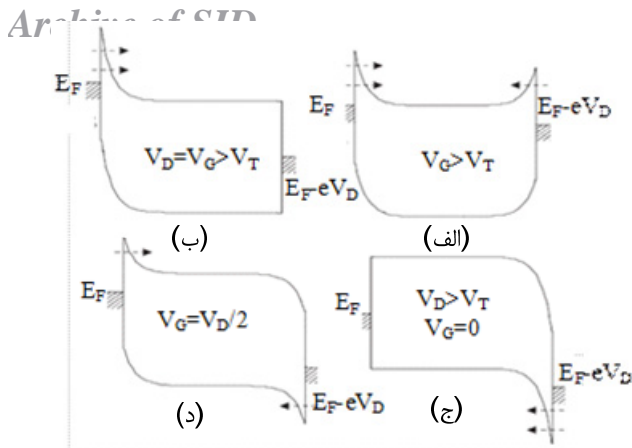
شکل ۳: دیاگرام باند انرژی SBGNRFET تحت بایاس مختلف [۱۷].
