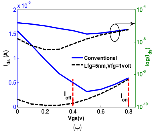
شکل ۶: مشخصه جریان-ولتاژ I_{DS}-V_{GS} ، (الف) در V_{DS}=0.6V و (ب) در V_{DS}=0.8V .
