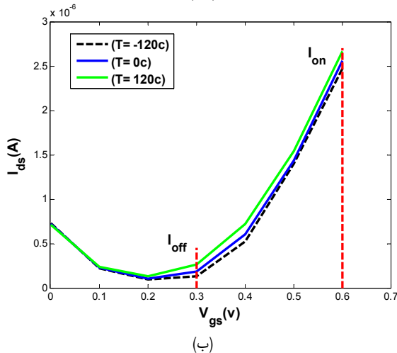
شکل ۱۰: مشخصه جریان-ولتاژ I_{DS}-V_{GS} در V_{DS} = 0.6V (الف) ترانزیستور متداول و (ب) ترانزیستور پیشنهادی با L_{FG} = 5nm و V_{FG} = 1V .
