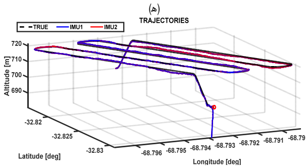
شکل ۷: روند مسیریابی سامانه‌های ناوبری بهینه‌سازی شده به واسطه بهترین اجرای الگوریتم‌های (الف) GA، (ب) PSO، (ج) IPO، (د) MIPO، (ه) SIPO و (و) HIPO در مقایسه با مسیر مرجع True.
