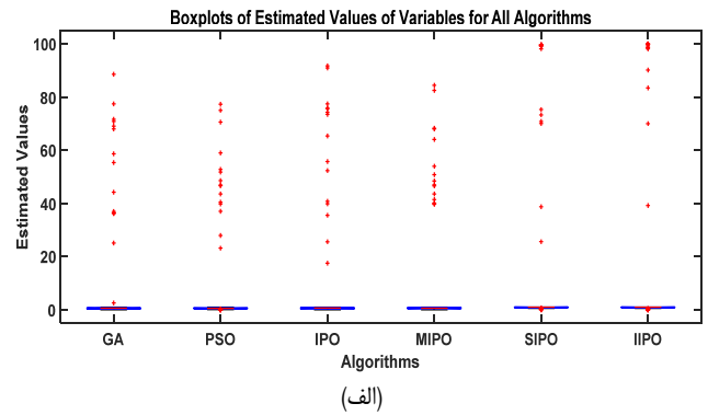
شکل ۵: نمودار جعبه‌ای متغیرهای طراحی در طول ۵ اجرای مستقل به ازای کلیه الگوریتم‌ها.
