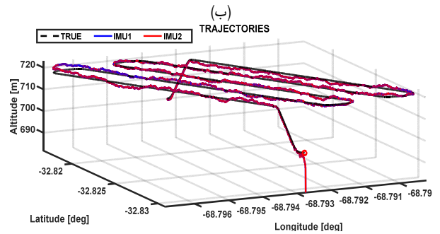
شکل ۷: روند مسیریابی سامانه‌های ناوبری بهینه‌سازی شده به واسطه بهترین اجرای الگوریتم‌های (الف) GA، (ب) PSO، (ج) IPO، (د) MIPO، (ه) SIPO و (و) HIPO در مقایسه با مسیر مرجع True.
