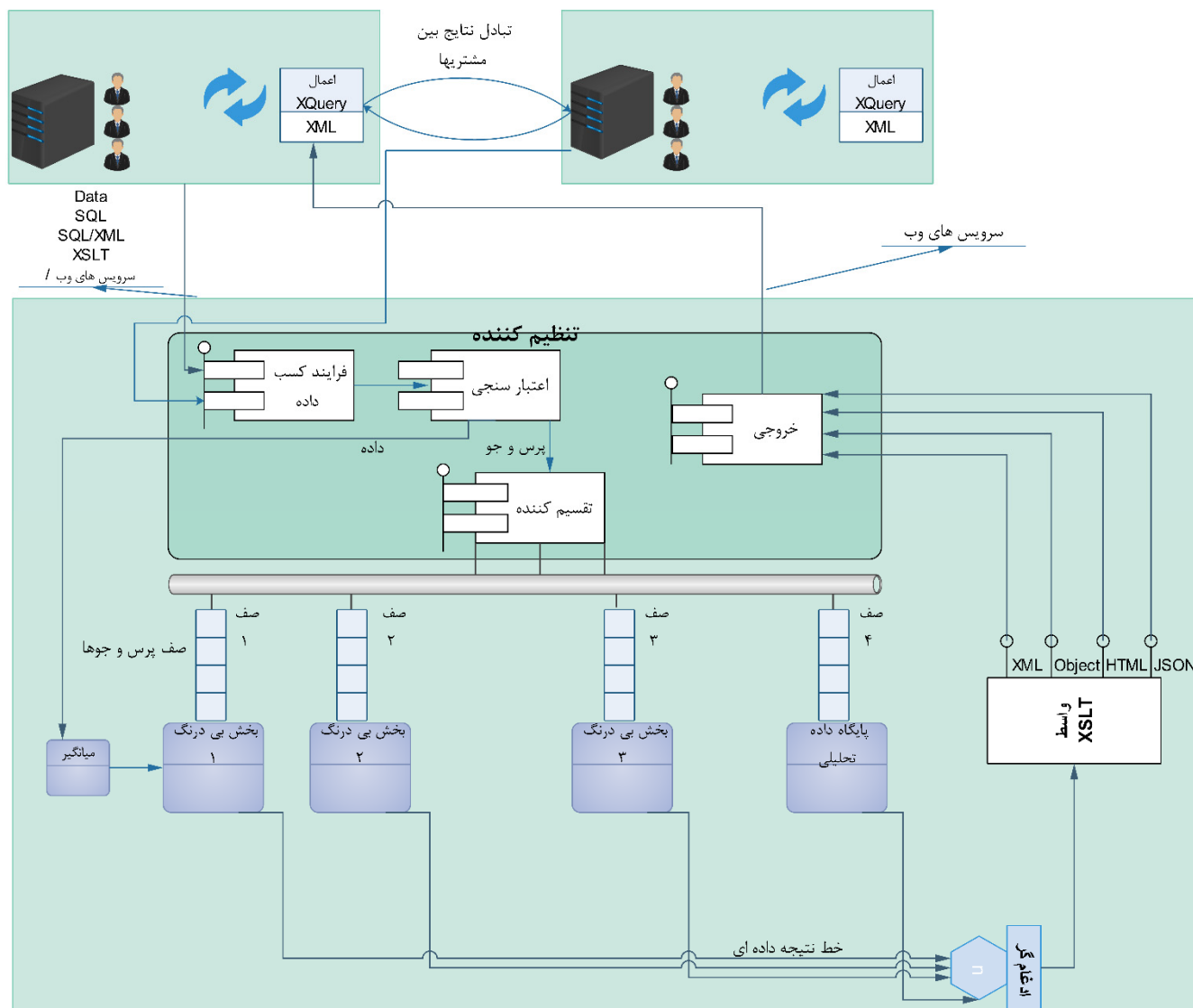
شکل ۱: معماری پیشنهادی.
