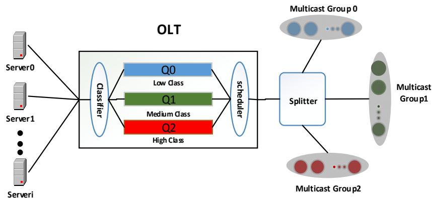
شکل ۱: معماری EPON برای روش FWA [۹].
