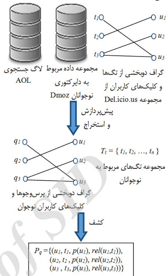
شکل ۴: روند کشف الگوی موضوعی کلیک‌های کاربران نوجوان به ازای هر پرس‌وجو.
