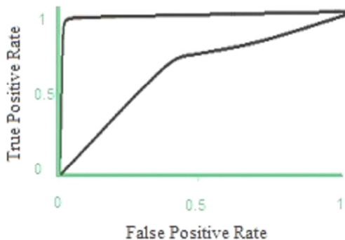
شکل ۸: منحنی ROC کلاسه‌بندی دودویی.
