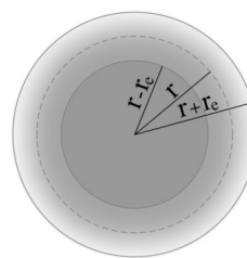
شکل ۱: شعاع حسگری یک گره با مدل حسگری احتمالی.
