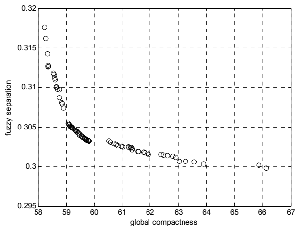
شکل ۲: جواب‌های بهینه پارتو در حالت FSIS در مجموعه داده Colon.
