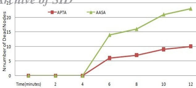
شکل ۱۰: تعداد گره‌های از دست رفته (مرده).
