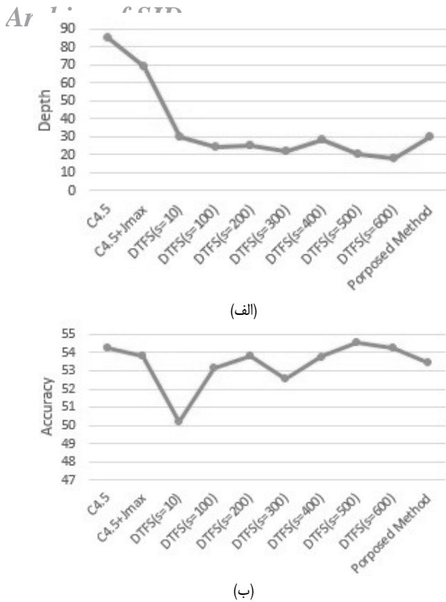
شکل ۳: (الف) عمق درخت تصمیم و (ب) دقت در درخت‌های تصمیم ساخته شده برای مجموعه داده Poker.
