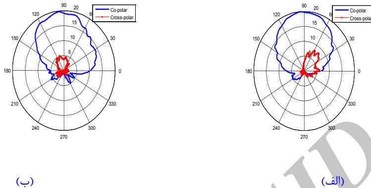
شکل ۵) نتایج اندازه گیری پترن تشعشی آنتن، (الف) صفحه E و (ب) صفحه H.
