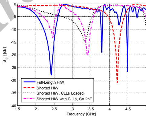
شکل (۱۱) افت بازگشتی، آنتن با ساختار HIW عمود بر خط تغذیه و اصلاح شده توسط ساختارهای CLL
