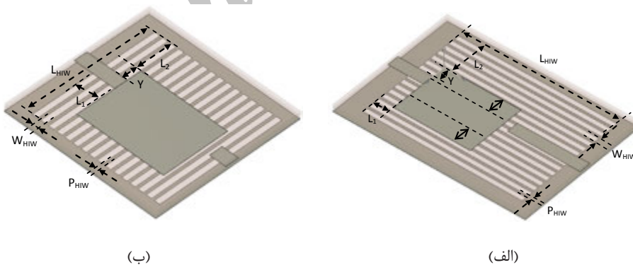
شکل ۶) ساختار آنتن در دو حالت ساختار HIW (الف) هم جهت با خط تغذیه و (ب) عمود بر خط تغذیه:
