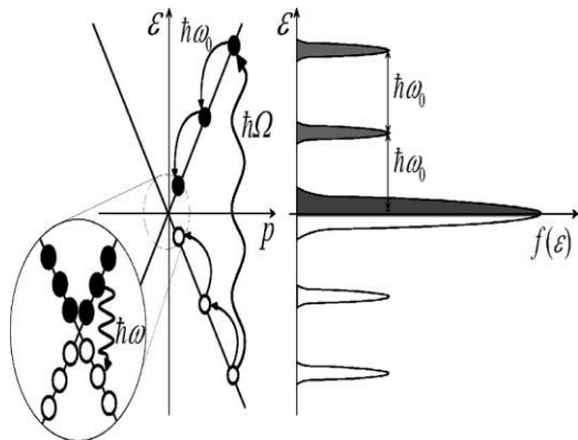
شکل ۲. دیاگرام باند و توزیع انرژی گرافن [۸]
