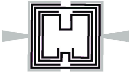
شکل ۴. سلول واحد تشدیدگر به همراه خط تغذیه (با رنگ خاکستری).
