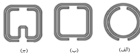
شکل ۱. حلقه‌های تشدید شکاف‌دار. الف) SRR دایروی، ب) SRR مربعی، ج) SRR با اصلاح طول [۱۱].
