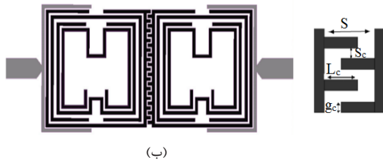
شکل ۱۱. الف) پارامترهای فیزیکی خازن بین‌انگشتی (ب) ساختار نهایی فیلتر شماره یک پیشنهادی.
