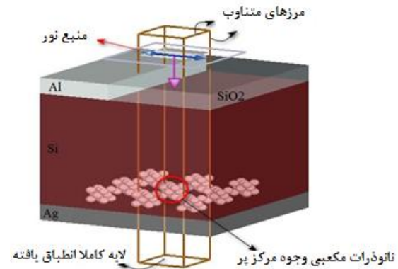
شکل ۵. سلول خورشیدی شامل نانو ساختارهای مکعبی و جوه مرکز پر
