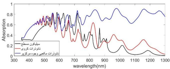
شکل ۷. نمودار مقایسه‌ای در سلول‌های خورشیدی
