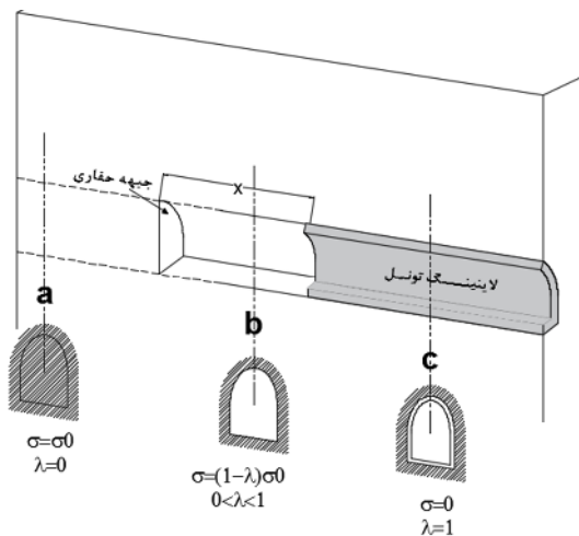
شکل ۲ - آزادی تنش در تونل (بر اساس González-Nicieza, Álvarez-Vigil, Menéndez-Díaz, & González-Palacio, 2008; Bernat & Cambou, 1998)
