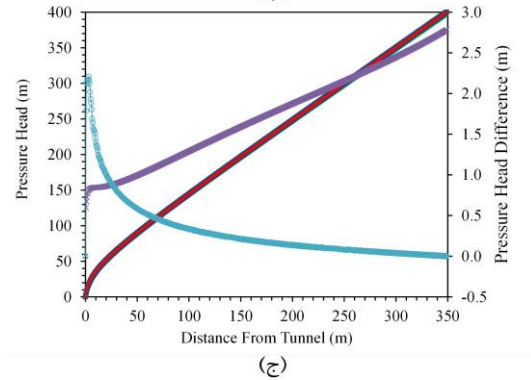
شکل ۷- مقادیر هد فشاری حاصل از سه روش کد محاسباتی FNETF ، نرم افزار Phase2 و حل تحلیلی (محور چپ) و اختلاف بین مقادیر هد فشاری حاصل از کد محاسباتی FNETF با دو روش دیگر (محور راست) بر روی خطوط شاخص: الف) L1، ب) L2، ج) L3
