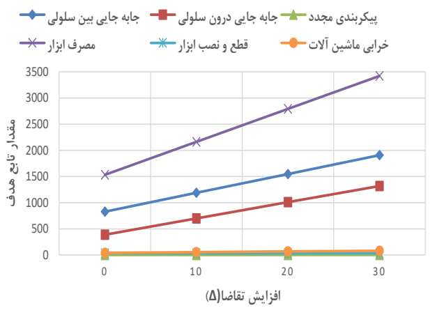
نمودار (۵): تاثیر افزایش تقاضا بر روی تابع هدف مدل
