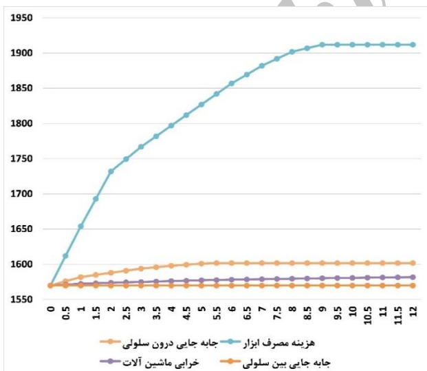
نمودار (۷): تأثیر افزایش پارامتر عدم قطعیت روی جابه‌جایی درون سلولی، بین سلولی، هزینه مصرف ابزار، خرابی ماشین‌آلات
