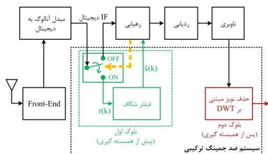
شکل (۲). سامانه ضدجمینگ پیشنهادی.
