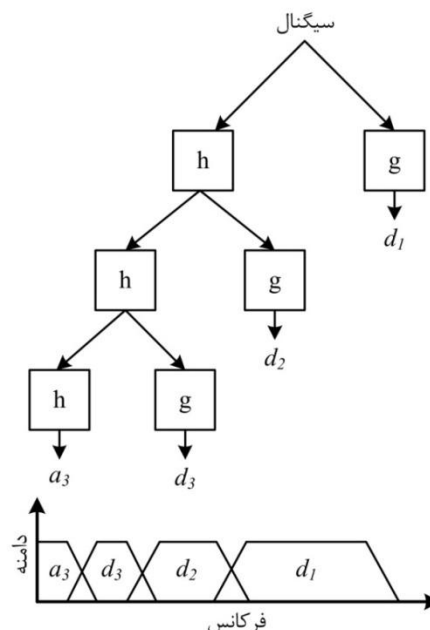
شکل (۱). تجزیه سیگنال به کمک DWT
