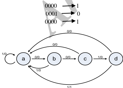
شکل (۵). دیاگرام حالت مکان صرفها در مدار آشکارساز کد
