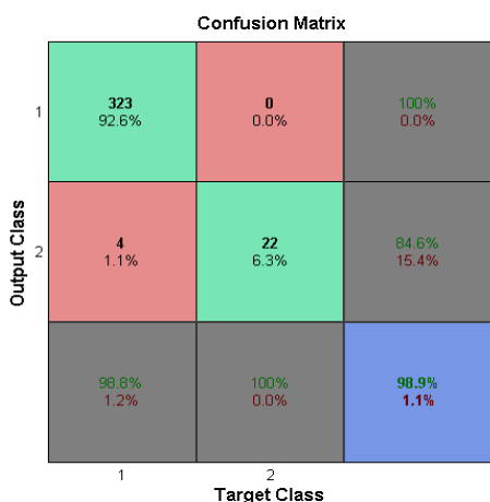
شکل (۱۵): ماتریس درهم‌ریختگی
