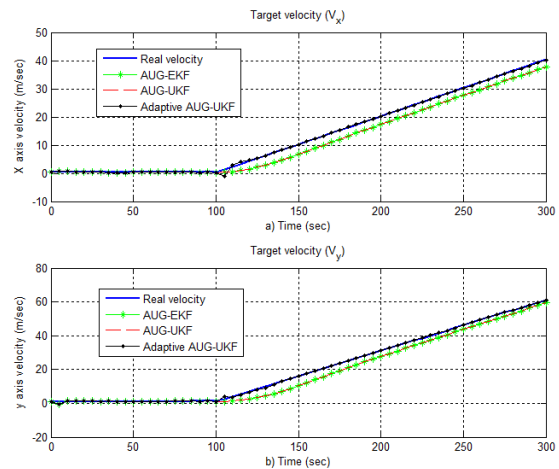
شکل (۳): نمودار سرعت واقعی هدف و تخمین های آن با روش پیشنهادی در مقایسه با روش های AUG-EKF و AUG-UKF در طول دو محور x و y در سناریو اول
