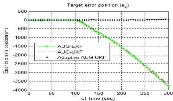
شکل (۷): جابجایی هدف در راستای محورهای x و y و تخمین روش پیشنهادی AUG-UKF تطبیقی در مقایسه با روش‌های AUG-EKF و AUG-UKF به همراه مقادیر خطای ردیابی در سناریوی شتاب متوسط هدف (سناریوی ۲)
