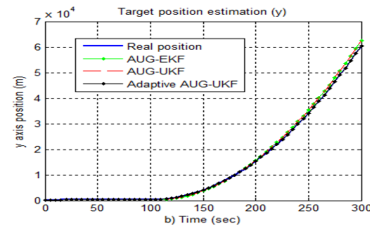
شکل (۶): تخمین مسیر حرکتی هدف با روش پیشنهادی در مقایسه با روش‌های AUG-EKF و AUG-UKF در سناریوی مانور کم (تصویر بزرگ‌نمایی شده)
