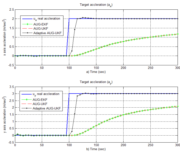
شکل (۹): نمودار شتاب‌گیری هدف در لحظه t = 100 (Sec) و t چگونه تخمین شتاب هدف با استفاده از روش پیشنهادی و مقایسه آن با دو روش AUG-UKF و AUG-EKF در سناریو دوم
