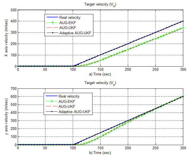
شکل (۸): نمودار سرعت واقعی هدف و تخمین‌های آن با روش پیشنهادی در مقایسه با روش‌های AUG-UKF و AUG-EKF در طول دو محور x و y در سناریو دوم
