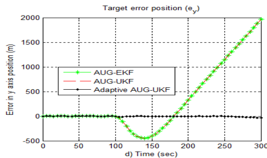
شکل (۷): جابجایی هدف در راستای محورهای x و y و تخمین روش پیشنهادی AUG-UKF تطبیقی در مقایسه با روش‌های AUG-EKF و AUG-UKF به همراه مقادیر خطای ردیابی در سناریوی شتاب متوسط هدف (سناریوی ۲)
