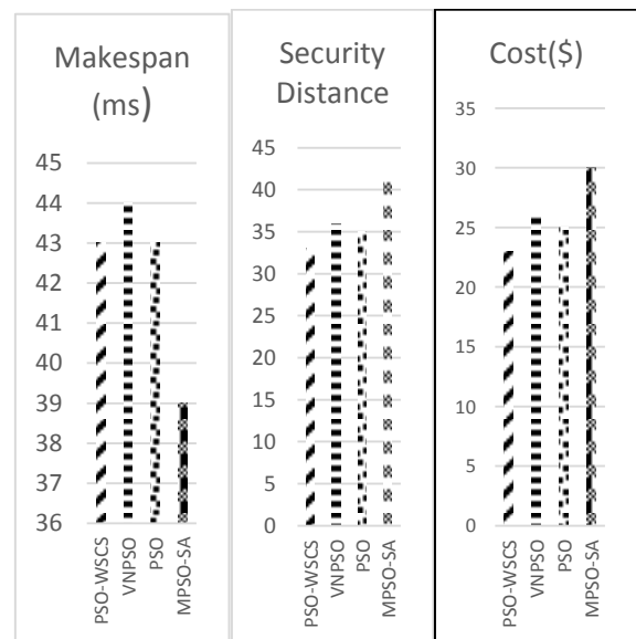
شکل (۸): تابع هدف، زمان اجرا و هزینه روی گراف HEFT
