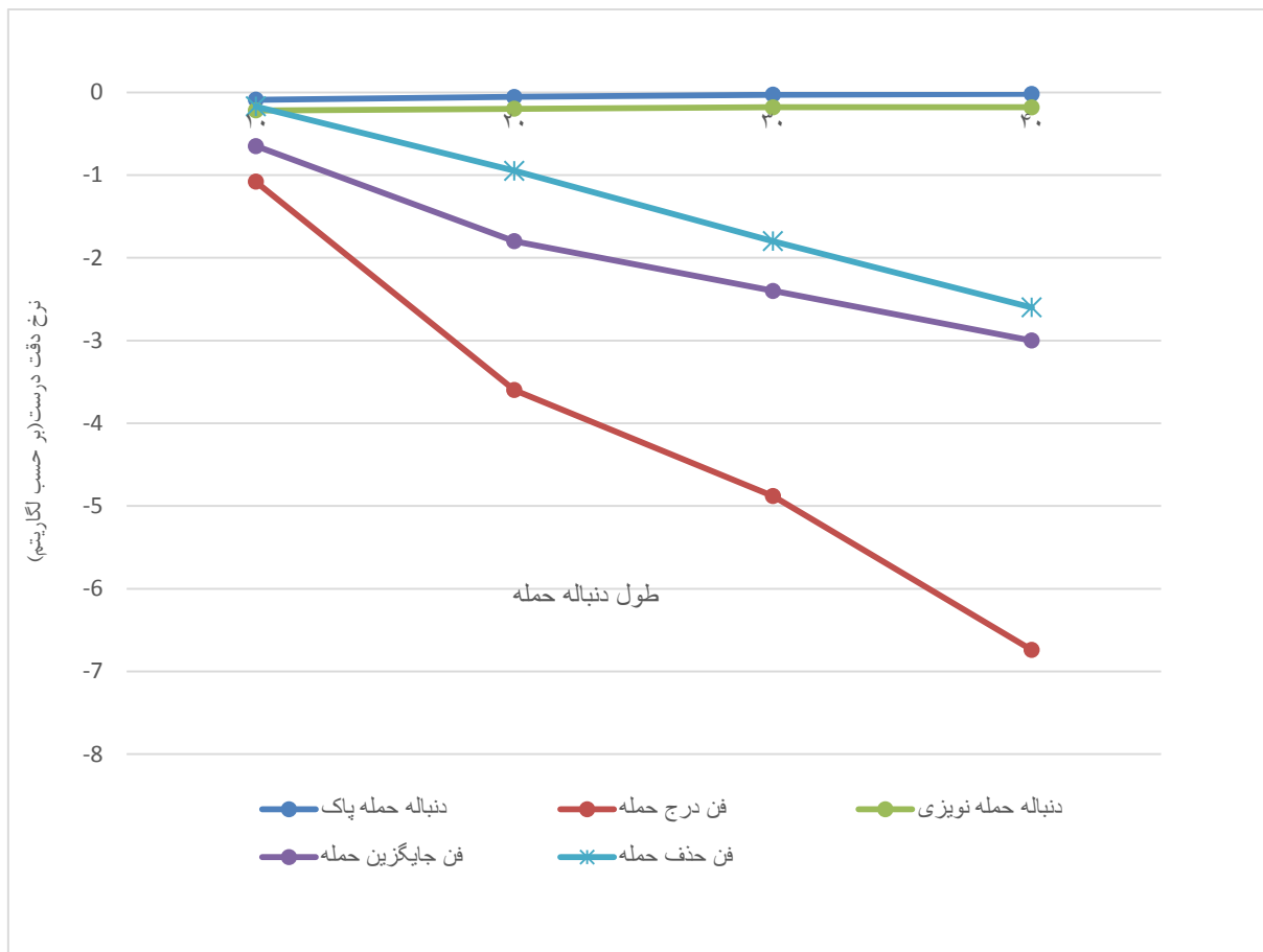
نمودار (۱): مقایسه دقت مبهم‌سازی مدل پیشنهادی برای فنون مختلف با حملات پاک
