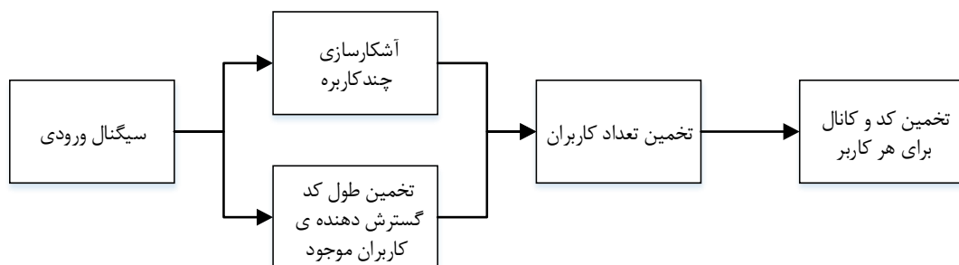
شکل (۱): نمودار قالبی سامانه شود چند کاربره طیف گسترده دنباله مستقیم
