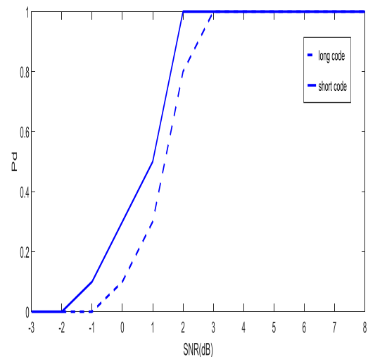
شکل (۷): مقایسه میان کدهای کوتاه و بلند در کانال AWGN
