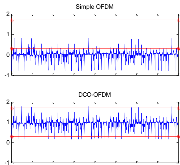
شکل (۱): اثر اضافه کردن DC بایاس به سمبل OFDM
