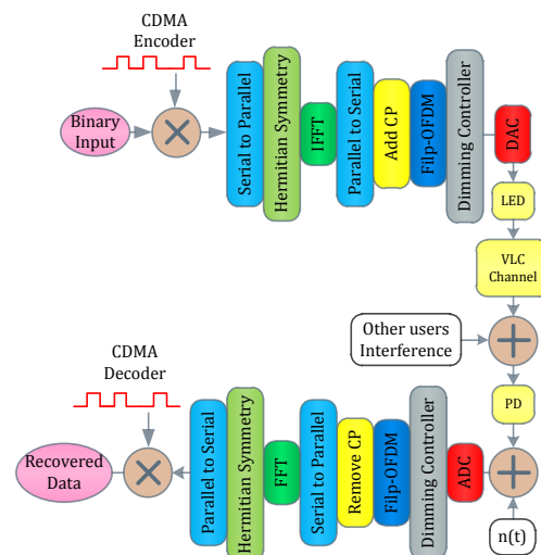
شکل (۲): بلوک دیاگرام سامانه OFDM-CDMA مبتنی بر VLC.
