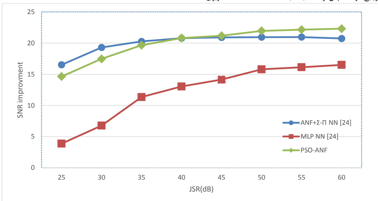
شکل (۶): نمودار میزان بهبود SNR الگوریتم پیشنهادی در مقایسه با سایر روش‌ها در حذف جمر تک فرکانس.
