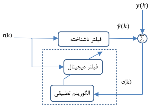
شکل (۲): بلوک دیاگرام فیلتر شکاف تطبیقی.
