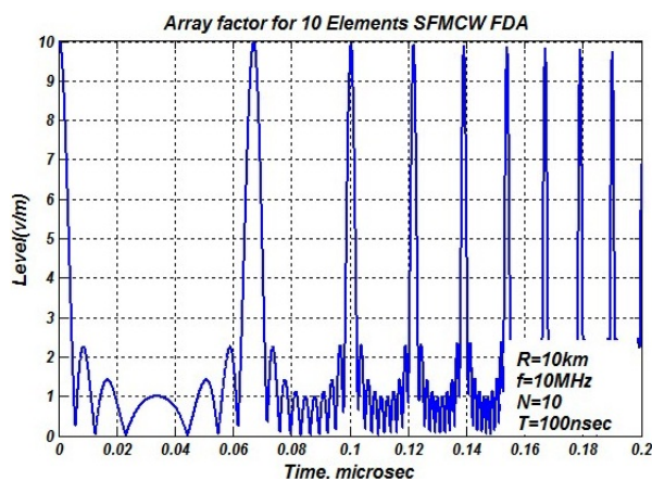
شکل ۶. الگوی تشعشی آرایه SFMCW نسبت به زمان در فاصله ثابت R=10km
