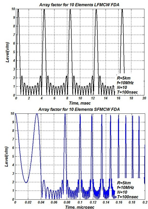
شکل ۱۰. مقایسه الگوی تشعشی FDA مبتنی بر SFMCW با FDA مبتنی بر LFM CW و مقایسه دوره تناوب آن‌ها نسبت به زمان
