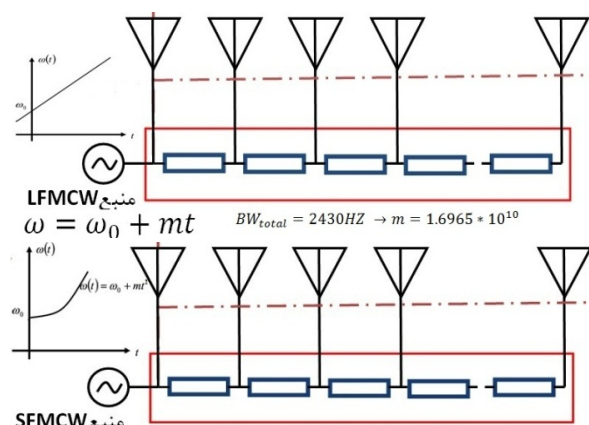
شکل ۸. ساختار آرایه FDA مبتنی بر SFMCW و آرایه FDA مبتنی بر LFM CW متناظر با آن
