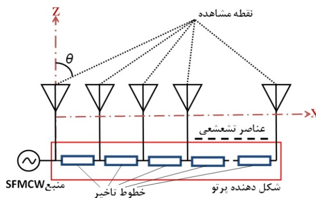
شکل ۳. ساختار آرایه با چندگانگی فرکانس مبتنی بر رژیم فرکانسی مرتبه دو
