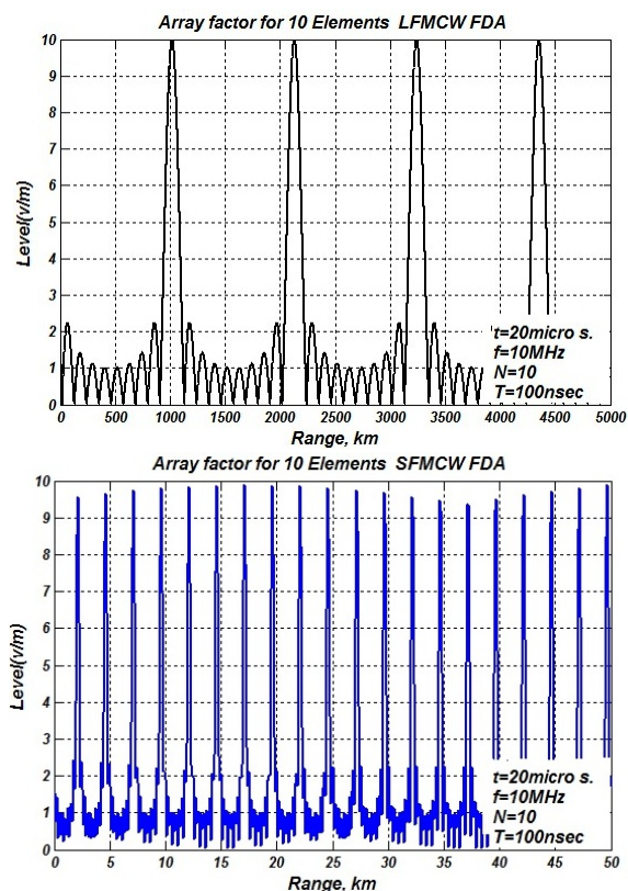
شکل ۹. مقایسه الگوی تشعشی FDA مبتنی بر SFMCW و آرایه FDA مبتنی بر LFM CW و مقایسه دوره تناوب آن‌ها نسبت به فاصله
