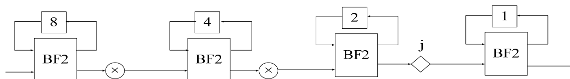
شکل ۵. معماری R2SDF برای FFT ۱۶ نقطه‌ای [۱۴]
