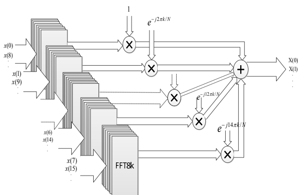
شکل ۸. نمایش FFT راستای سمت به صورت FFT های ۸۱۹۲ نقطه‌ای
