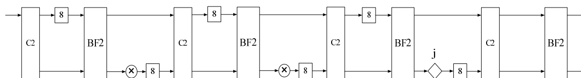
شکل ۵. معماری R2MDC برای FFT ۱۶ نقطه‌ای [۱۳]
