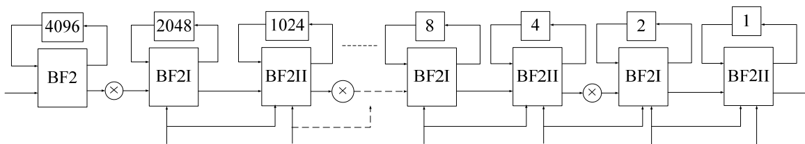
شکل ۱۰. ساختار هسته‌ی FFT ۸۱۹۲ نقطه‌ای
