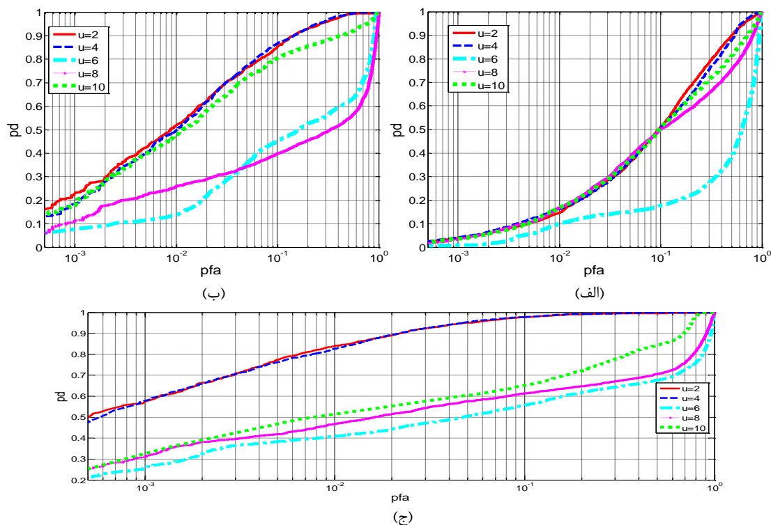
شکل ۵. تعیین ضریب مناسب \frac{\sigma_{bpdn}}{\sigma} در حالت آشکارسازی در راستای بُرد به‌ازای پارامترهای جدول ۳. الف) SNR = 0 dB، ب) SNR = \Delta dB، ج) SNR = \lambda dB
