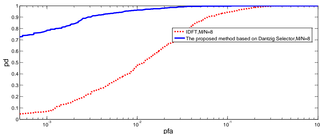
شکل ۱۵. نمودار ROC برای هدف با سرعت v=20m/s و نرخ M/N=8 برای روش IDFT و روش حسگری فشرده مبتنی بر Dantzig Selector
