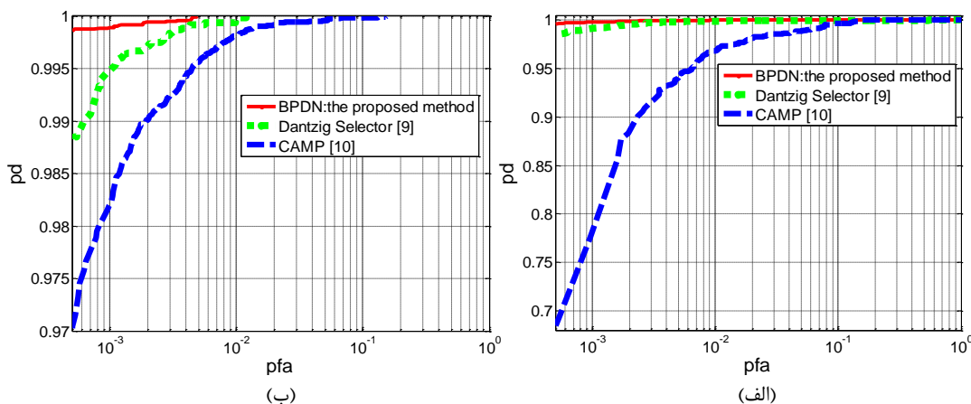
شکل ۶. مقایسه روش ۲D-BPDN با روش ارائه‌شده در [۱۰-۱۱] در حالت آشکارسازی در راستای بُرد. پارامترهای این شکل متناظر با جدول ۴ هستند. الف) N = 80 ، ب) N = 120
