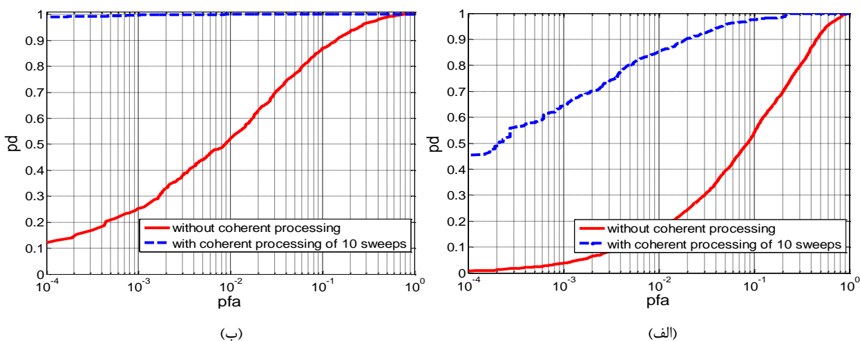
شکل ۱۰. تأثیر انتگرال‌گیری همدوس روی نمودار ROC. پارامترهای شکل متناظر با جدول ۵ هستند. الف) K=5 و SNR=0\text{dB} ، ب) K=50 و SNR=5\text{dB} .
