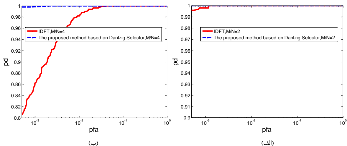
شکل ۱۴. نمودار ROC برای هدف با سرعت v=20m/s در روش IDFT و روش حسگری فشرده مبتنی بر Dantzig Selector (الف) M/N=2 و (ب) M/N=4
