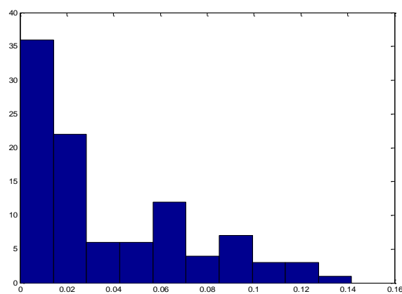
شکل ۱۱. تابع چگالی احتمال D_e تست کولموگروف-اسمیرنوف برای داده‌های با پارامترهای تخمین‌زده با روش پیشنهادی در آزمایش یک
