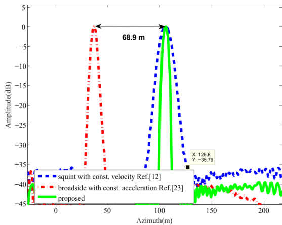
شکل ۸. تابع PSF در جهت سمت یک هدف تحت زاویه لوچی سه درجه با استفاده از روابط پیشنهادی (خط توپر)، روابط جانب نگر (خط نقطه) و لوچ با سرعت ثابت (خط چین)
