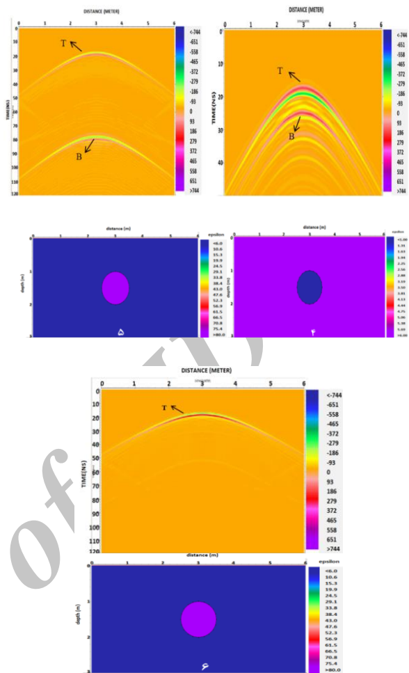
شکل (۱۰): بررسی تأثیر نوع سیال محتوی هدف استوانه‌ای روی پاسخ GPR. مدل ۴: استوانه توخالی، مدل ۵: استوانه پر از آب شیرین، مدل ۶: استوانه پر از آب شور
