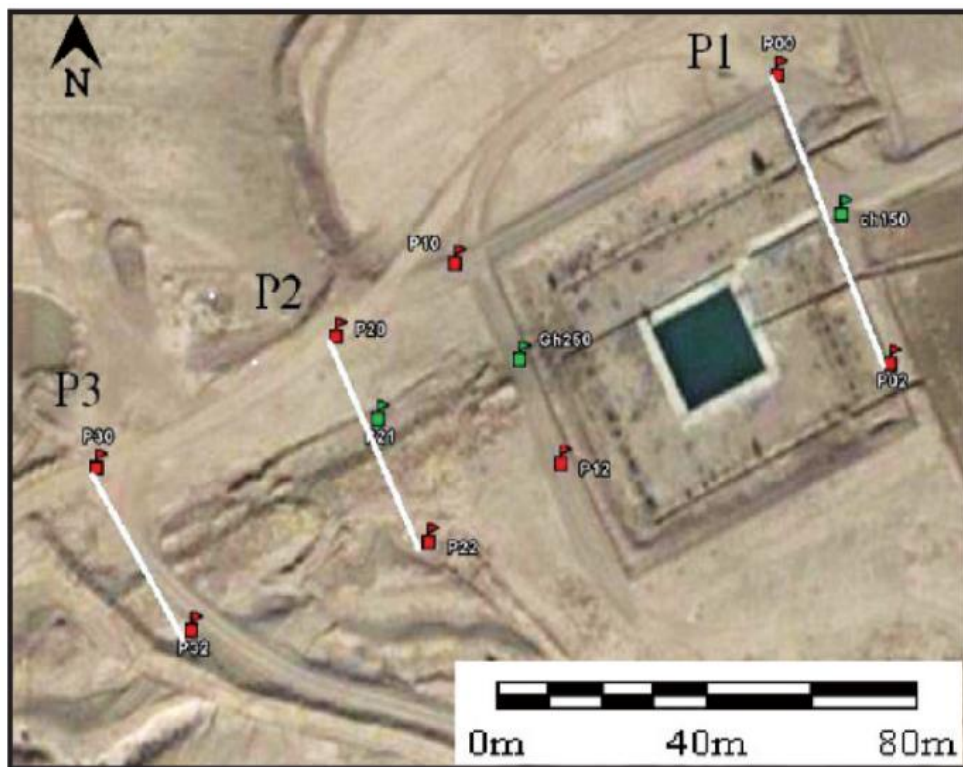
شکل (۱۴): عکس هوایی منطقه برداشت به همراه پروفیل‌های برداشتی و نقاط اندازه‌گیری مختصات مکانی (GPS) برگرفته از سایت Google Earth [۲۴].
