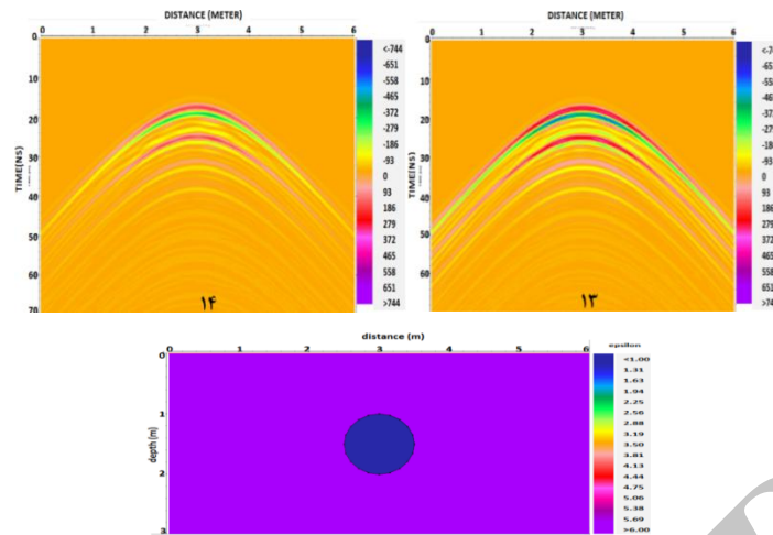
شکل (۱۲): بررسی تأثیر رسانندگی الکتریکی محیط میزبان روی پاسخ GPR دو هدف استوانه‌ای. برای مدل ۱۳: \sigma_h = 0.1 \text{ mS/m} و برای مدل ۱۴: \sigma_h = 10 \text{ mS/m} محیط میزبان و ۰: هدف.
