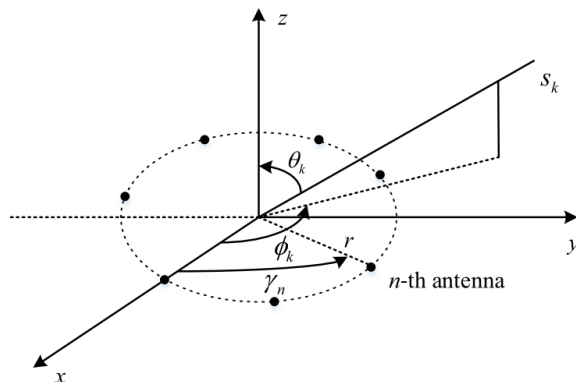
شکل (۱): آرایه دایروی یکنواخت با N آنتن.
