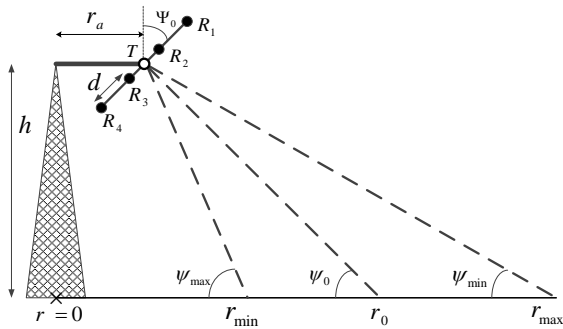
شکل (۶): هندسه تصویربرداری و آرایه
