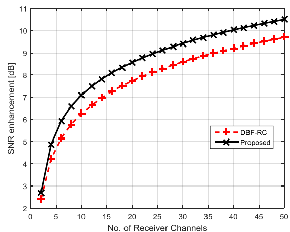
شکل (۱۲): مقدار افزایش SNR نسبت به حالت تک‌کانال بر حسب تعداد کانال گیرنده در برد دور (زاویه برخورد 67/5 درجه)
