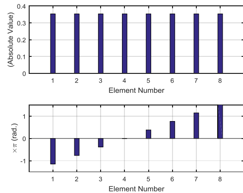
شکل (۱۱): اندازه و فاز ضرایب وزن‌دهی کانال‌های گیرنده در روش DBF-RC برای برد دور (زاویه برخورد 67/5 درجه)
