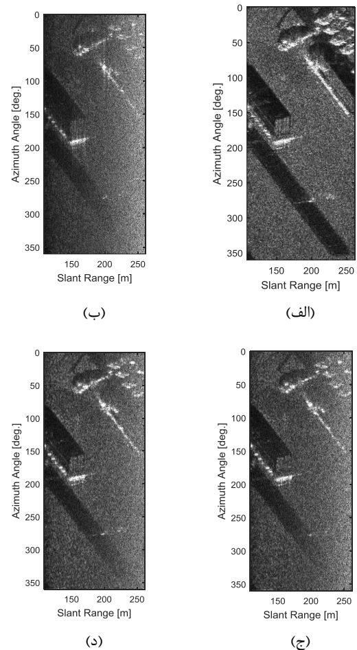
شکل (۱۳): تصویر صحنه بر حسب زاویه سمت و برد مایل: (الف) تصویر اولیه، (ب) تصویر با استفاده از یک کانال گیرنده، (ج) تصویر با استفاده از روش DBF-RC و (د) تصویر با استفاده از روش پیشنهادی
