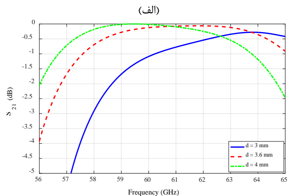
شکل (۷): ضرایب انتقال و انعکاس مبدل مود TE_{10} موجبر مستطیلی به مود TM_{01} موجبر دایروی به ازای مقادیر مختلف d .
