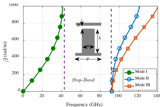
شکل (۳): نمودار پاشندگی ساختار متناوب از پین‌های فلزی. ابعاد برحسب میلی‌متر عبارتند از: a = 0.5 , h = 1 , p = 1 و g = 0.2 .
