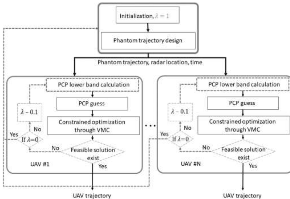
شکل (۴): بلوک دیاگرام طراحی مسیر برای پهپادهای همکار جهت فریب شبکه راداری. در قسمت اول مسیر هدف مجازی طراحی می‌شود. این مسیر می‌تواند به کمک بهینه‌سازی محاسبه شود و یا به صورت پیش فرض در نظر گرفته شود. در بخش دوم ابتدا با توجه به مسیر هدف مجازی، حد پایین مؤلفه طراحی مسیر محاسبه می‌شود و سپس مسیر حرکت پهپادها طراحی می‌شود. در صورت نبود پاسخ قابل قبول برای مسیر پهپادها، از مقدار \lambda کاسته می‌شود. در صورتی که به ازای \lambda = 0 پاسخ قابل قبول وجود نداشت، مسئله جهت اصلاح مسیر هدف مجازی و یا ارتقاء پهپادها به بخش اول ارجاع می‌شود. قسمت‌های خط چین، نوآوری این پژوهش را نشان می‌دهد.
