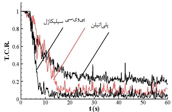
شکل (۱۱): مقایسه اختلاط ذرات شن ۲۷۵ میکرومتری با سه نوع ردیاب مختلف.
