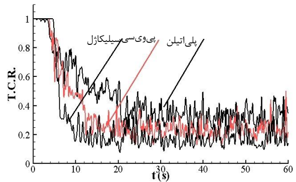
شکل (۱۰): مقایسه اختلاط ذرات شن ۴۶۰ میکرومتری با سه نوع ردیاب مختلف.
