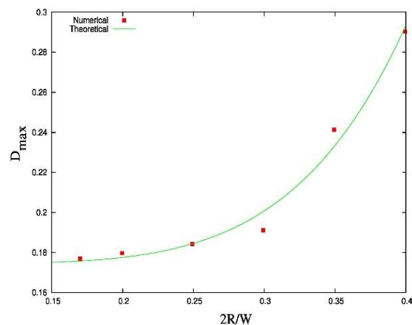
شکل (۲): بیشینه تغییر شکل یک گلبول قرمز برحسب اندازه گلبول. پارامترهای عددی: Ca_m = 0.81 و \mu = 3 .
