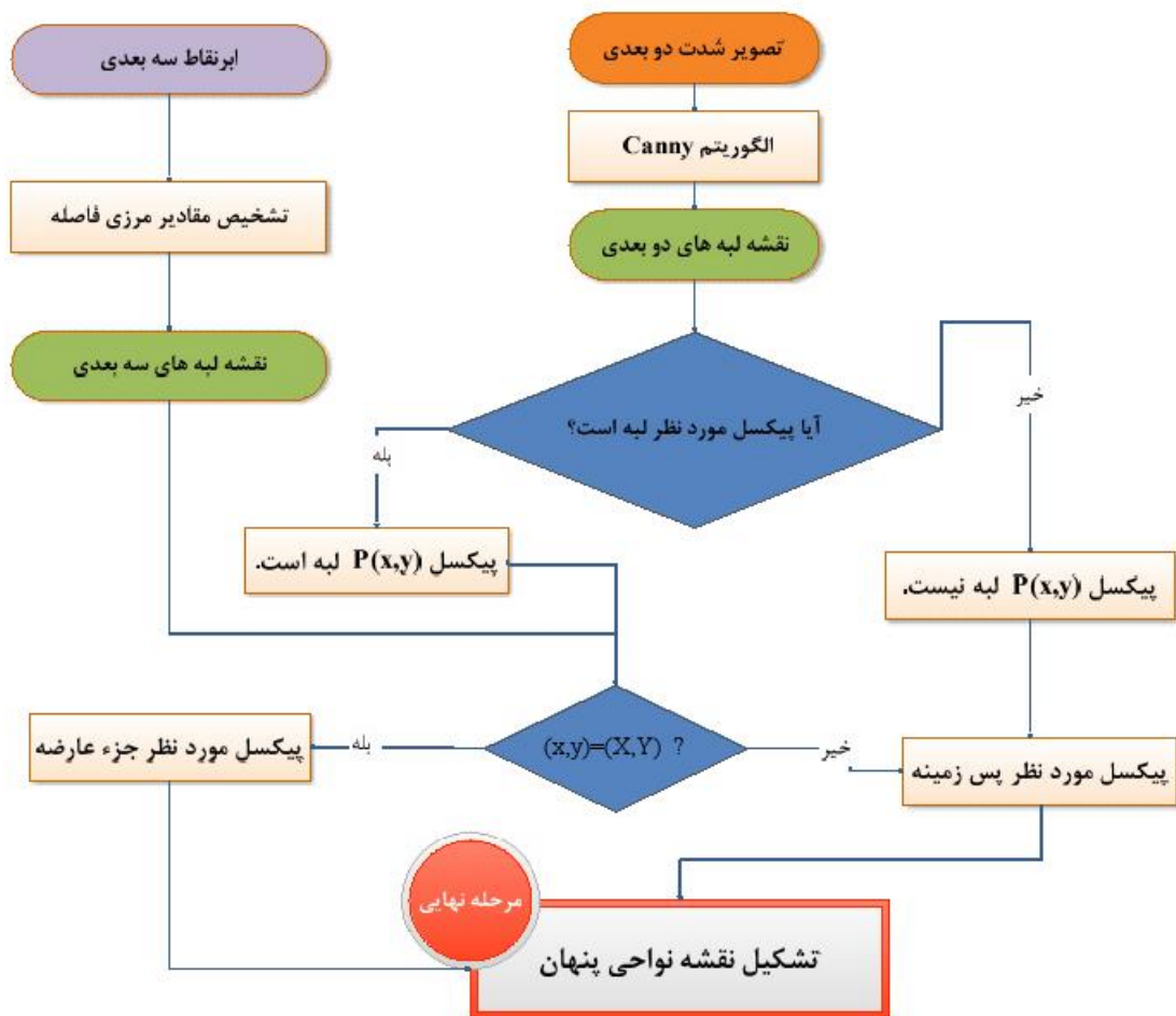
شکل ۶: فرآیند ترکیب لبه های دو بعدی و سه بعدی استخراج شده به منظور تشکیل نواحی پنهان
