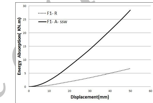
شکل ۲۵- منحنی جذب انرژی قاب‌های F1-R و F1-A-SSW
