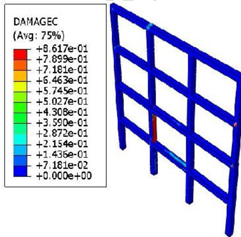
شکل ۱۶- خردشدگی فشاری بتن در قاب دارای دیوار برشی فولادی F1-A-SSW
