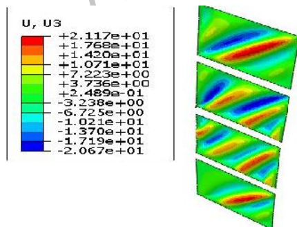
شکل ۲۴- نمایی از میدان پس کمانش ورق در تغییر مکان حداکثر بام برابر ۵۰ میلی متر
