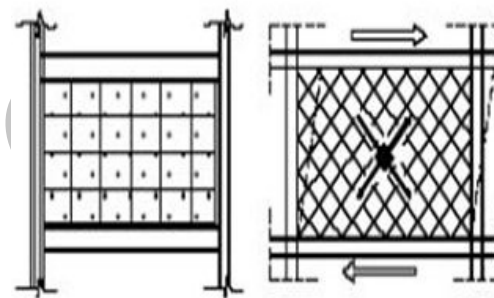
مکانیزم برشی خالص (پانل تقویت شده)
