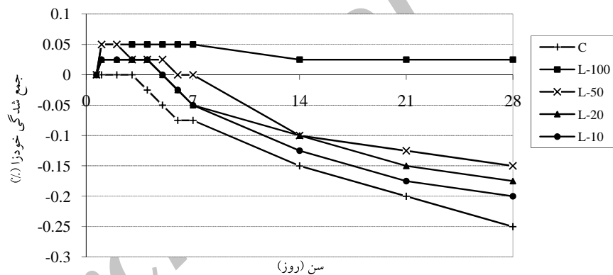
شکل ۲- جمع شدگی خودزایی ملات های سیمانی
