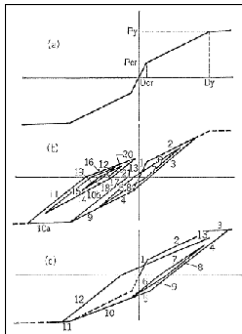
شکل ۴- منحنی هیستریزس بتن (Takeda) [۱۹]
