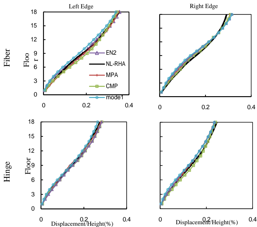
شکل ۱۰- نسبت جابجایی کف‌ها به ارتفاع سازه، حاصل از آنالیزهای بار افزون MPA، CMP، EN2، Model1 و تحلیل NL-RHA در لبه‌های نرم و سخت ساختمان نامتقارن در پلان از نوع TF.
