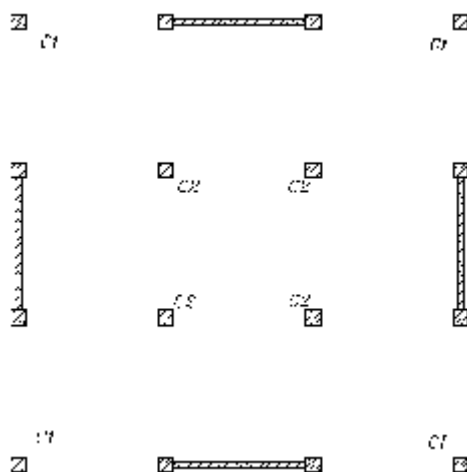
شکل الف-۱ پلان تپ بندی ستون ها
