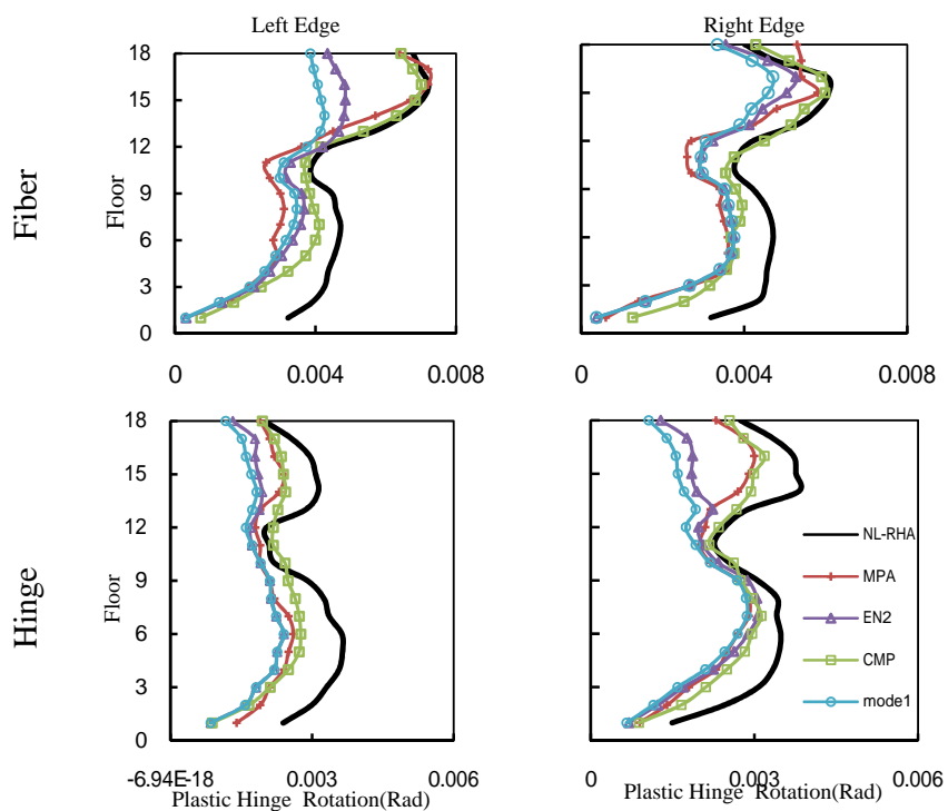
شکل ۱۶- دوران پلاستیک مفاصل، حاصل از آنالیزهای بار افزون MPA، CMP، EN2، Mode1 و تحلیل NL-RHA در
