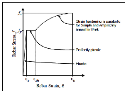
شکل ۵- منحنی تنش کرنش فولاد (Park) [۲۰]
