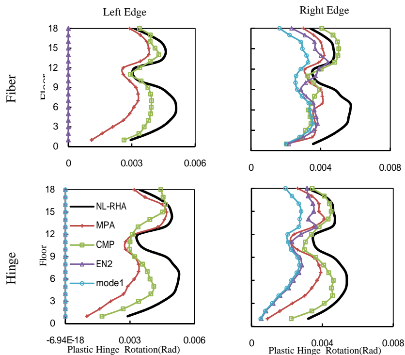
شکل ۱۵- دوران پلاستیک مفاصل، حاصل از آنالیزهای بار افزون MPA، CMP، EN2، Mode1 و تحلیل NL-RHA در
