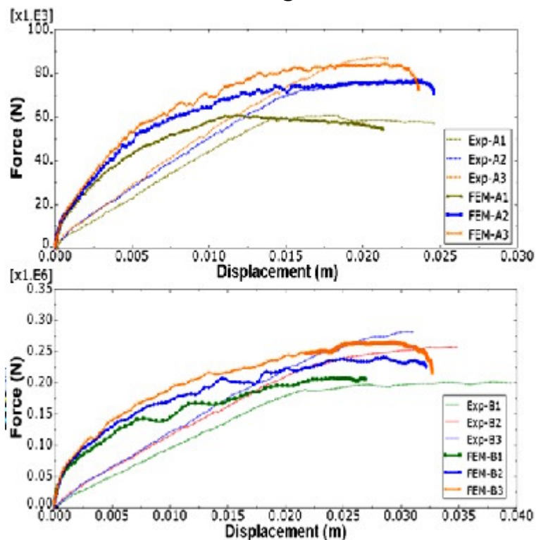
شکل ۱۱- منحنی نیرو-جابجایی (تغییر مکان وسط دهانه) تیرهای گروه A و B
