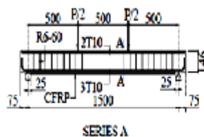
شکل ۱- جزییات مقاطع برای گروه‌های A و B [۲]
