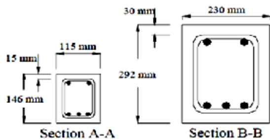
شکل ۱- جزییات مقاطع برای گروه‌های A و B [۲]
