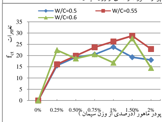
شکل ۵- مقاومت کششی نمونه های بتن حاوی پودر ماهور / شکل ۶- تغییرات مقاومت کششی بتن حاوی پودر ماهور
