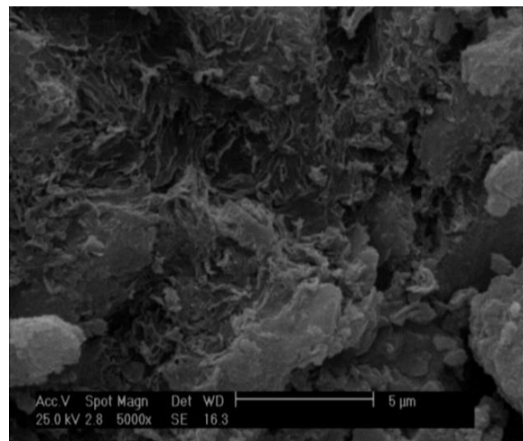
شکل ۱۶: تصویر میکروسکوپ الکترونی با مقیاس 5 \mu\text{m} از نمونه با عیار سیمانی ۳۰۰ و نسبت آب به سیمان ۰,۵ (تصویر سمت چپ نمونه بدون زئولیت و تصویر سمت راست نمونه با ۱۵ درصد زئولیت جایگزین سیمان).
