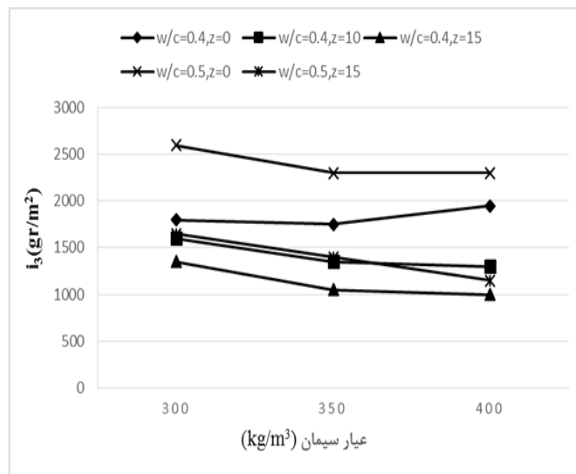
شکل ۶- نتایج جذب آب موئینه (۳ ساعت)
