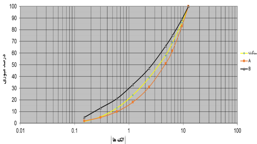
شکل ۱- منحنی سنگدانه مصرفی.
