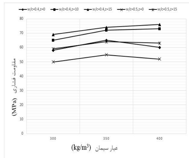
شکل ۲- نتایج آزمایش مقاومت فشاری ۲۸ روزه.
