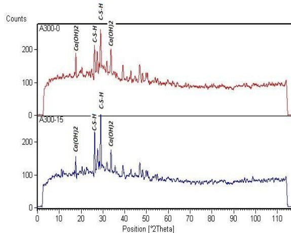
شکل ۱۱- طیف پراش پرتو ایکس نمونه های A300-15 و A300-0
