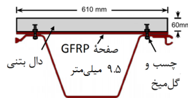
مقطع تیر دارای دال بتنی
