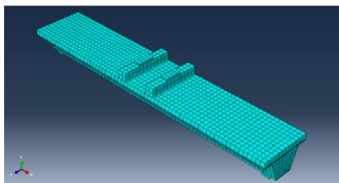
شکل (۴): مش‌بندی تیر کامپوزیتی
