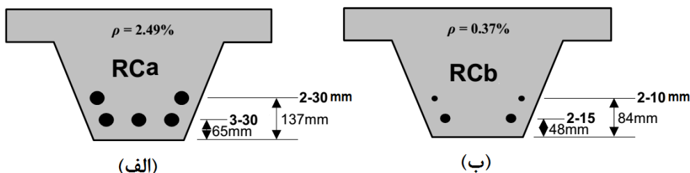
شکل (۱۷): مقطع تیر بتن مسلح (RC)؛
