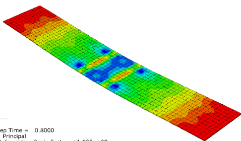
شکل (۱۲): تنش‌های اصلی فشاری صفحه GFRP در مدل عددی
