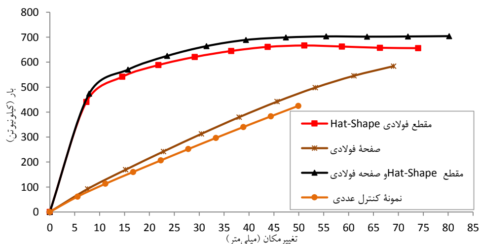
شکل (۲۰): نمودار بار - تغییر مکان مقطع Hat-Shape و صفحه GFRP به فولاد
